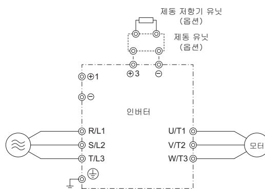
그림 3.5 주회로 단자의 연결
