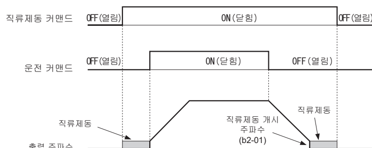
그림 5.69 직류제동의 타임차트
