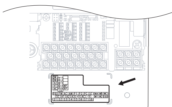
단자대의 아래 (CIMR-A□2A0110~2A0211, 4A0072~4A0165)
