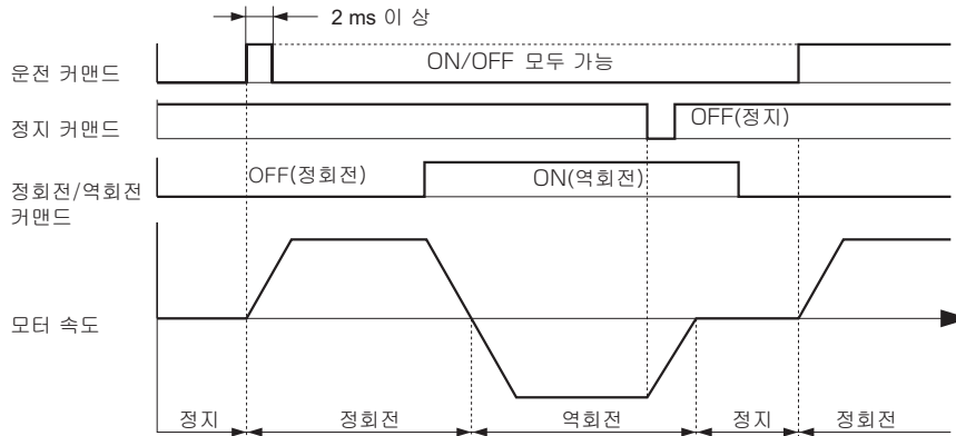
그림 5.62 3 와이어 시퀀스의 타임차트
