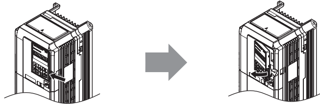
그림 3.19 오퍼레이터의 분리
