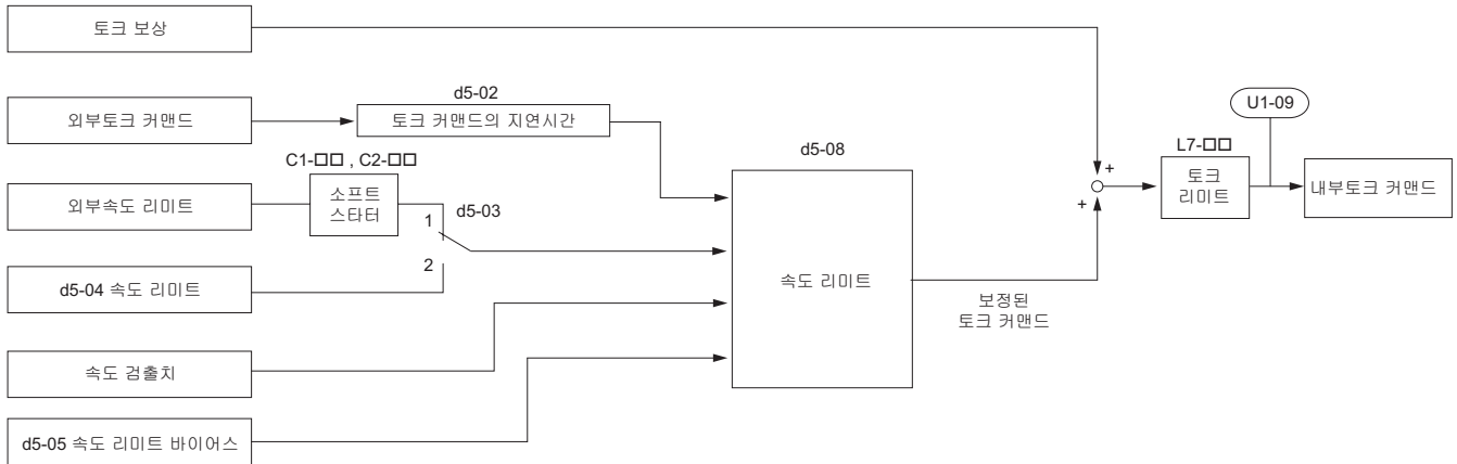
그림 5.53 토크제어 블록도
