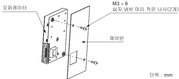
그림 2.6 제어반의 외측에 설치하는 경우
