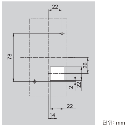
그림 2.7 제어반 가공 치수(제어반의 외측에 설치하는 경우)
