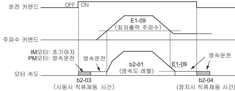
그림 5.14 영속운전
