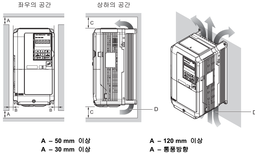
그림 2.2 인버터의 설치 공간(개체)
