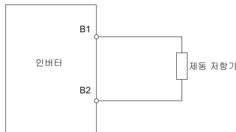
그림 8.11 제동 저항기의 연결(ERF형)
