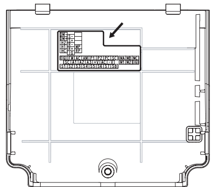
터미널 커버의 안쪽 (CIMR-A□2A0004~2A0081, 4A0002~4A0044)
