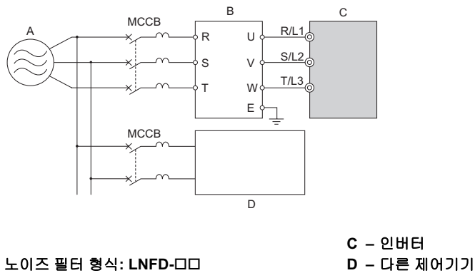
그림 8.19 입력측(1차측) 노이즈 필터의 연결 예
