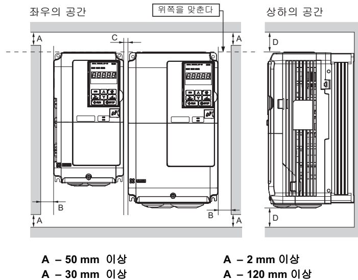
그림 2.3 인버터의 설치 공간( SIDE BY SIDE 설치)
