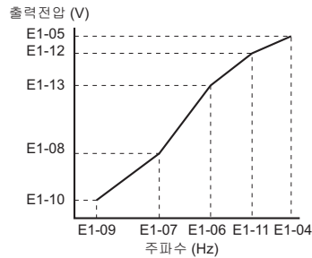
그림 5.56 V/f 패턴도
