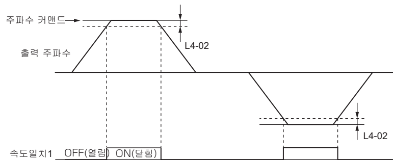
그림 5.73 속도일치 1의 타임차트
