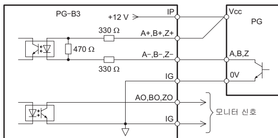
그림 8.7 인터페이스 회로도(오픈 콜렉터형)
