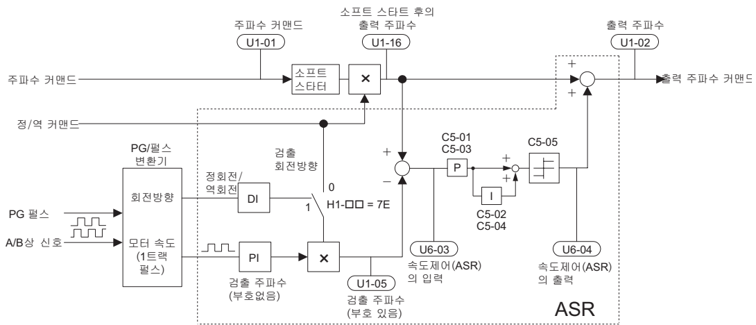
그림 5.93 간이 PG 장착 속도제어 블록도
