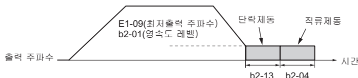
그림 5.16 정지시 단락제동(PG 미장착: PM 모니터)
